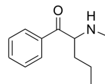
Pentedrone
