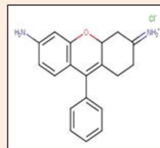
Rhodamine B
