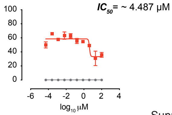
E64-d
