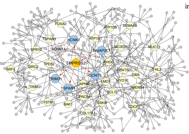
a. Colon UC BGRN
