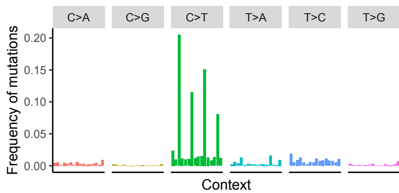
SIA4 (SBS17a+b - 0.93)
