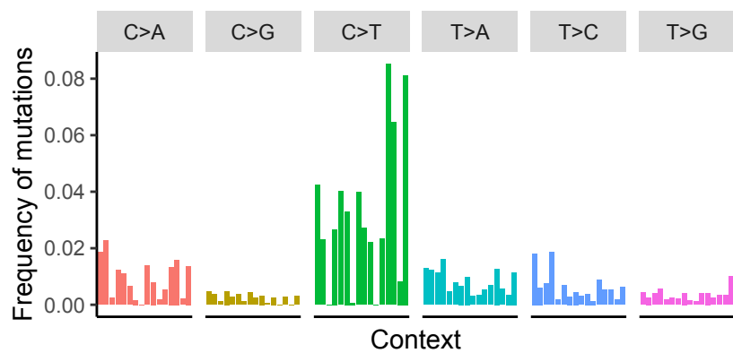
SIA7 (SBS30 - 0.81)
