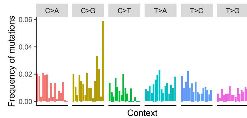
SIA6 (SBS26 - 0.89)
