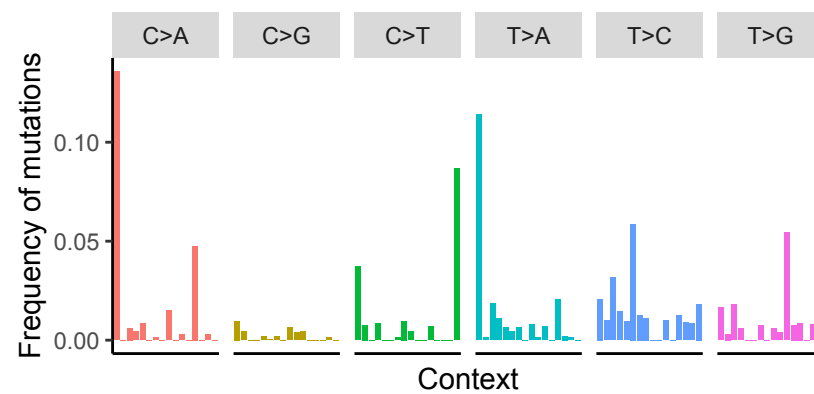
SIA8 (SBS51 - 0.93)
