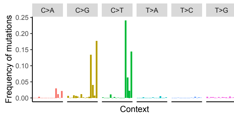
SIA5 (SBS18 - 0.89)
