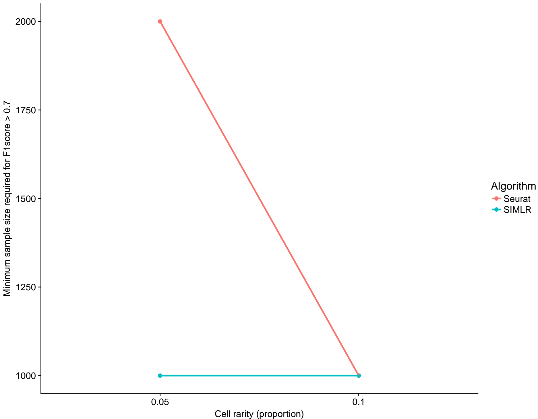
fC2, F1-score > 0.7
