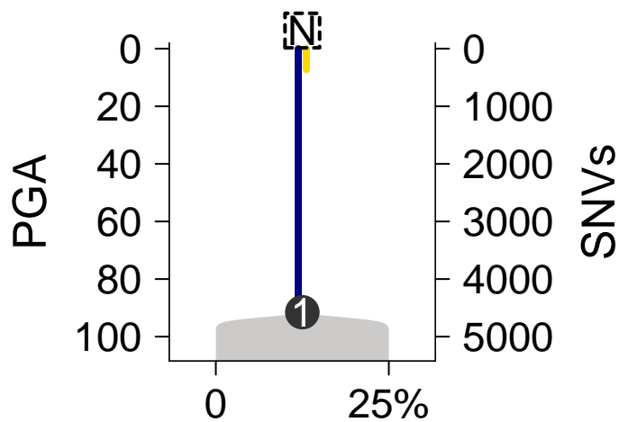
MuTect-TITAN
