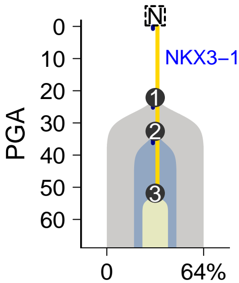
MuTect-Battenberg
