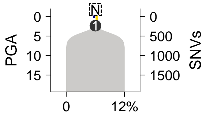
MuTect-TITAN
