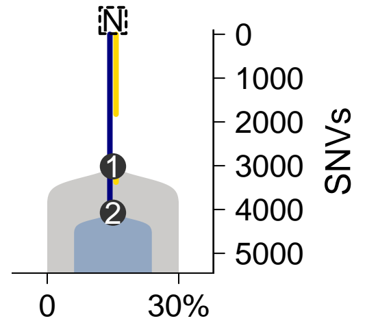
MuTect-TITAN
