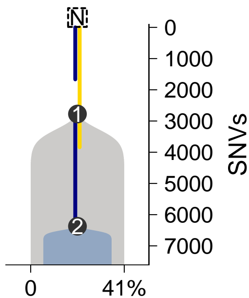
MuTect-TITAN
