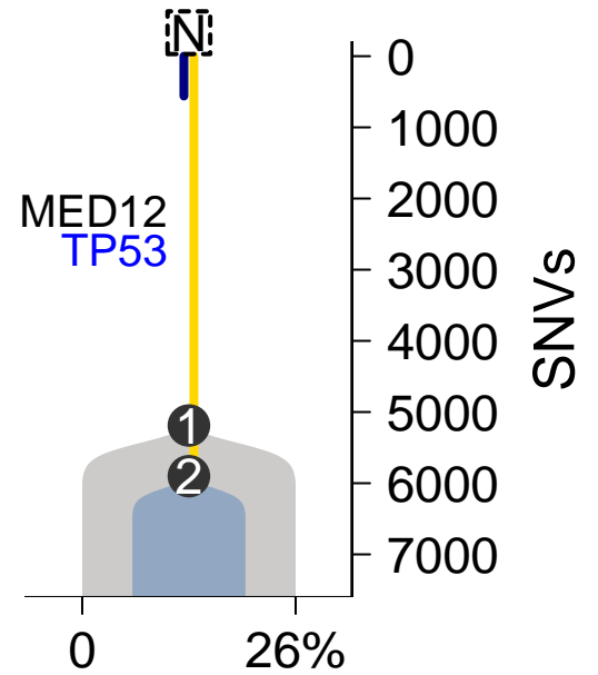
MuTect-TITAN
