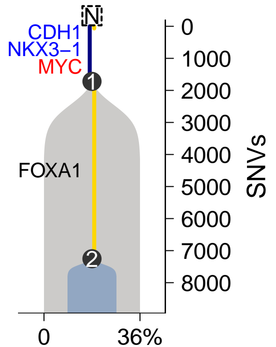
MuTect-TITAN
