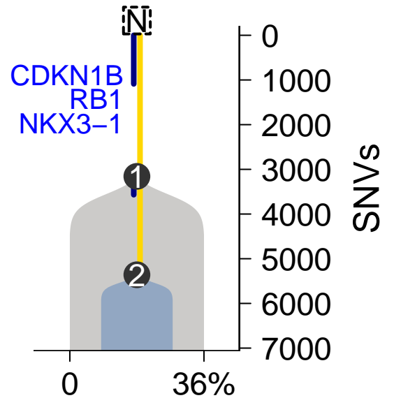
MuTect-TITAN
