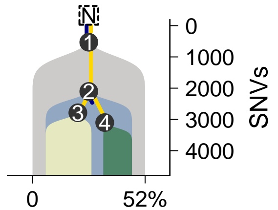
MuTect-TITAN
