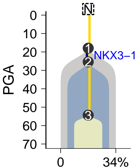
MuTect-Battenberg
