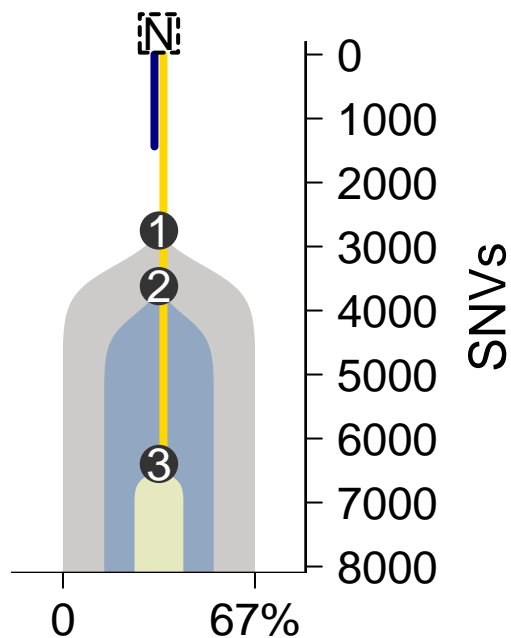
MuTect-TITAN
