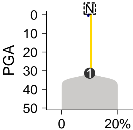
MuTect-Battenberg
