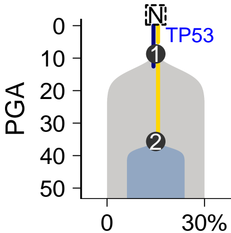
MuTect-Battenberg
