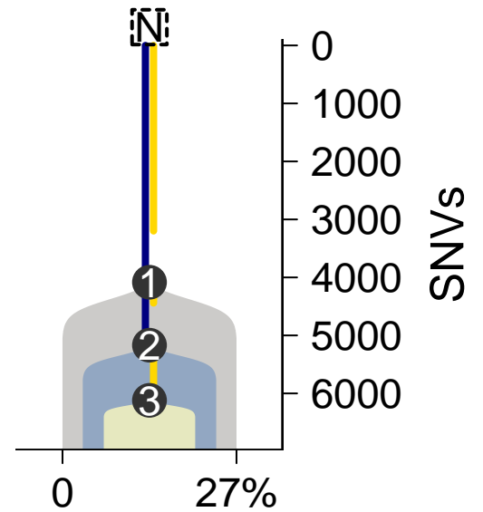
MuTect-TITAN
