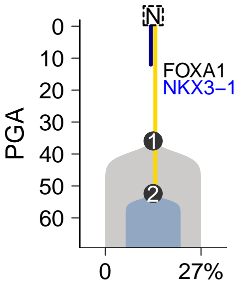
MuTect-Battenberg
