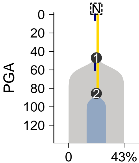
MuTect-Battenberg
