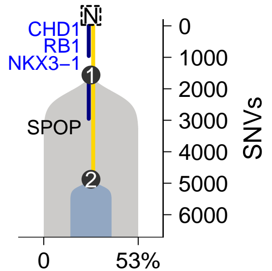
MuTect-TITAN
