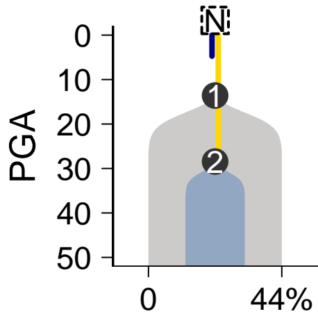
MuTect-Battenberg
