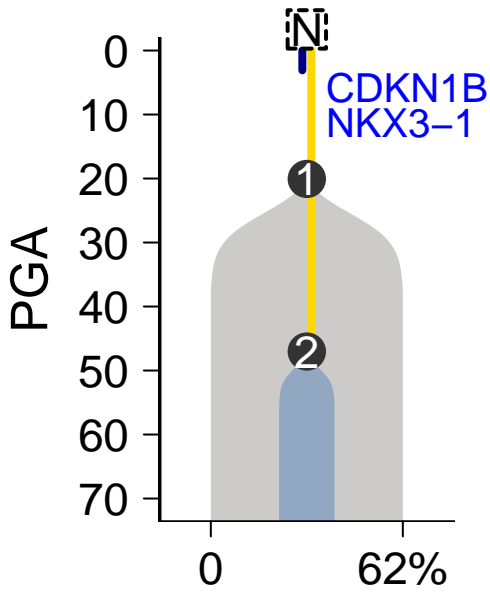
MuTect-Battenberg
