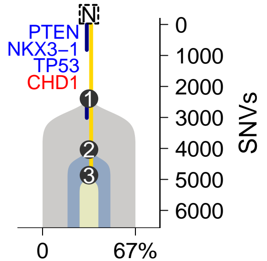
MuTect-TITAN
