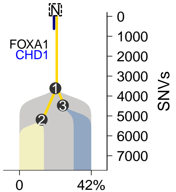
MuTect-TITAN
