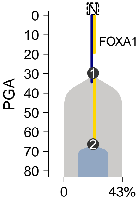
MuTect-Battenberg
