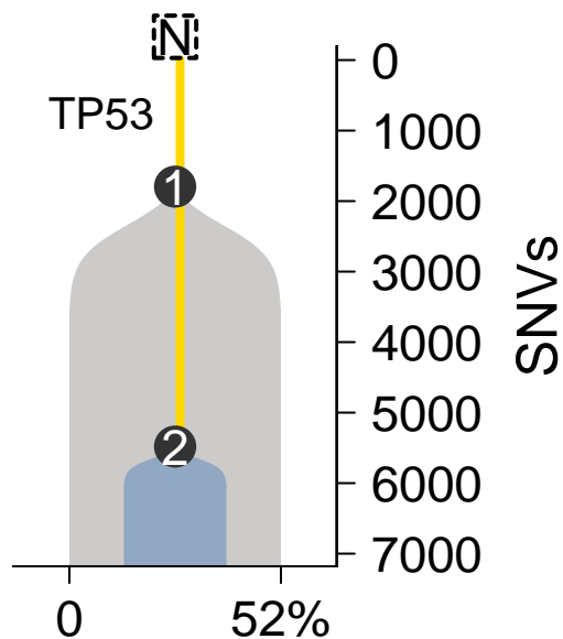
MuTect-TITAN
