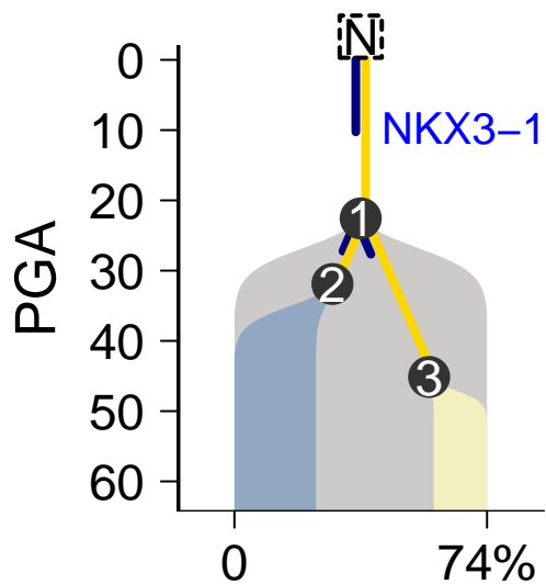
MuTect-Battenberg
