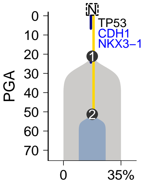
MuTect-Battenberg
