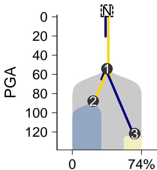
MuTect-Battenberg
