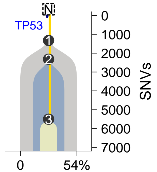
MuTect-TITAN
