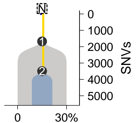
MuTect-TITAN
