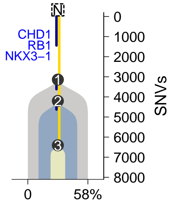
MuTect-TITAN
