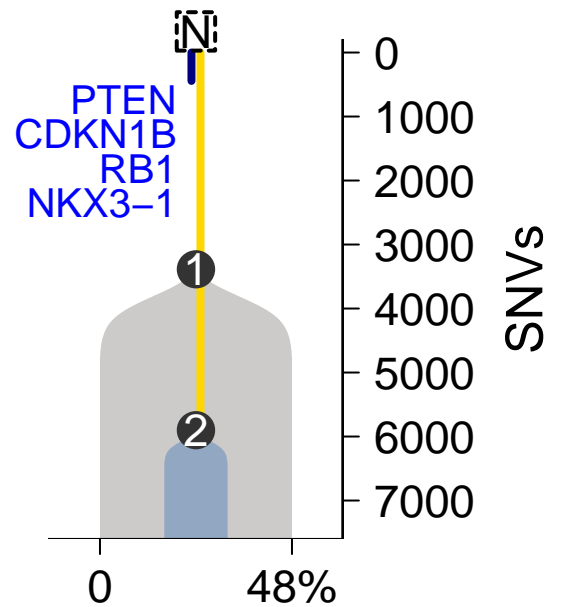
MuTect-TITAN
