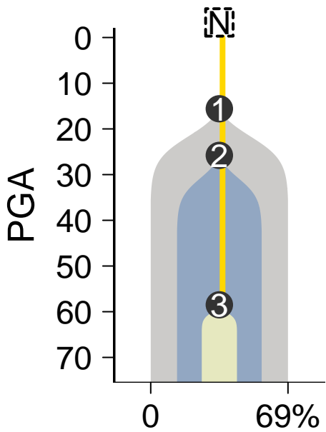
MuTect-Battenberg
