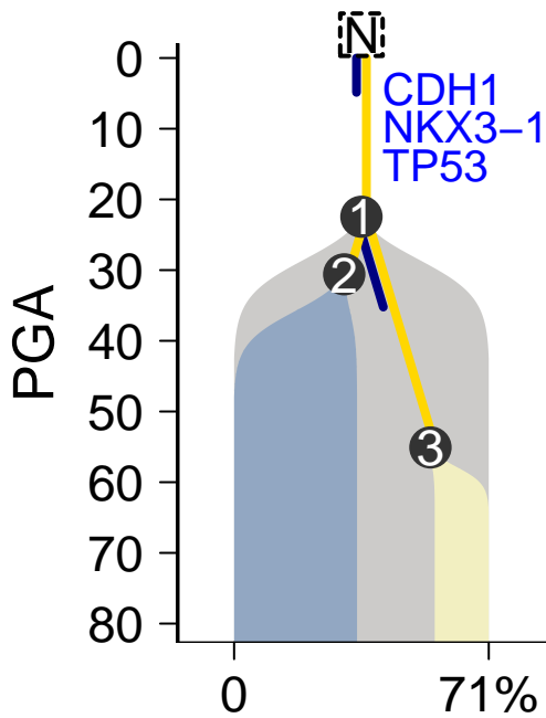
MuTect-Battenberg
