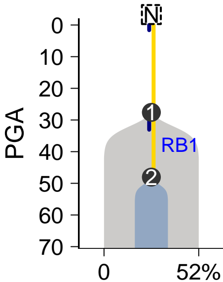
MuTect-Battenberg
