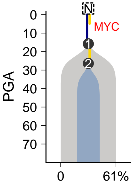
MuTect-Battenberg
