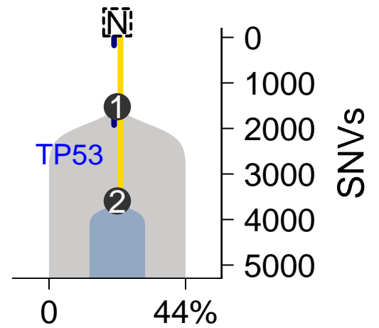
MuTect-TITAN
