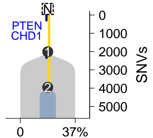
MuTect-TITAN
