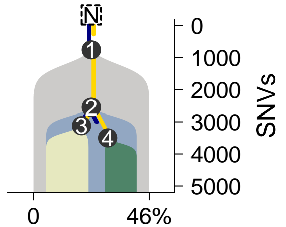
MuTect-TITAN
