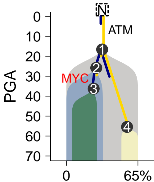
MuTect-Battenberg
