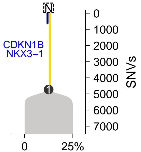
MuTect-TITAN
