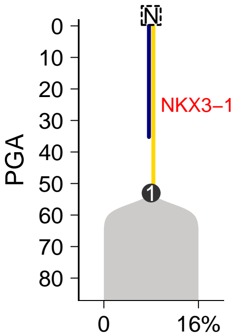
MuTect-Battenberg
