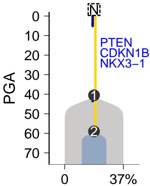
MuTect-Battenberg
