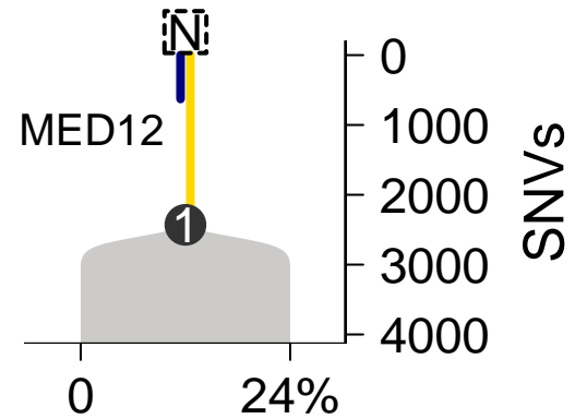
MuTect-TITAN
