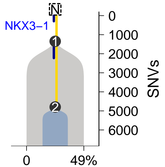
MuTect-TITAN
