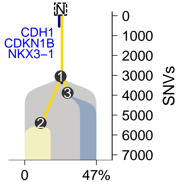
MuTect-TITAN
