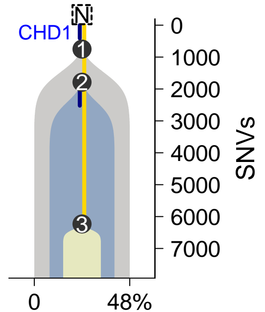
MuTect-TITAN
