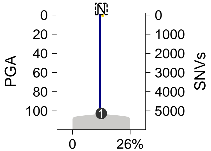
MuTect-TITAN
