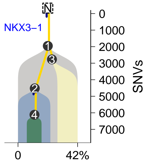
MuTect-TITAN
