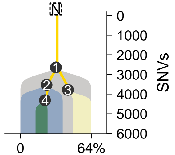
MuTect-TITAN
