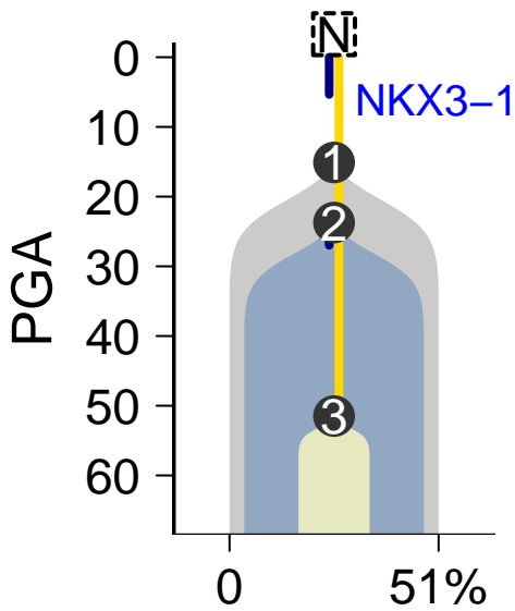
MuTect-Battenberg
