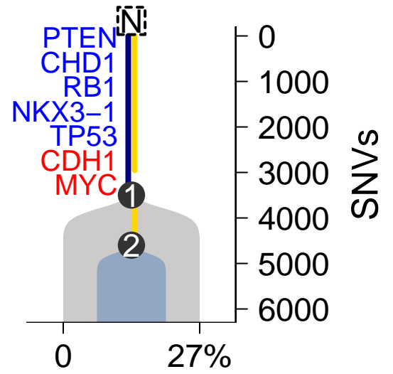
MuTect-TITAN
