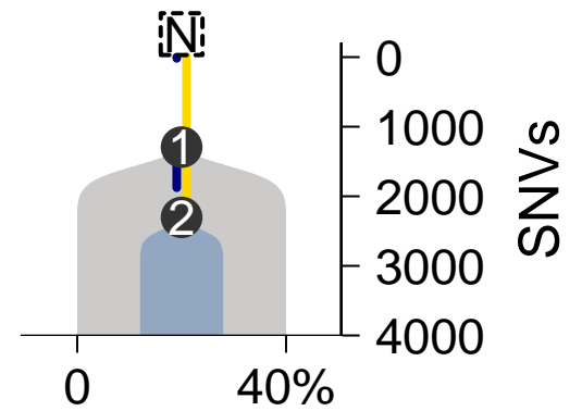
MuTect-TITAN
