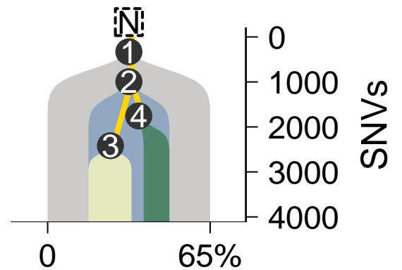
MuTect-TITAN
