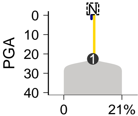
MuTect-Battenberg
