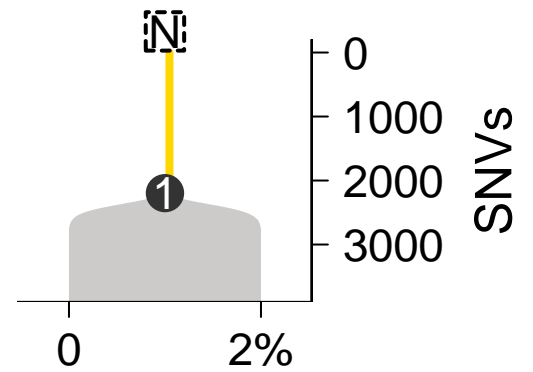
MuTect-TITAN
