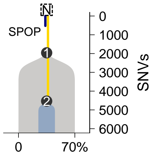
MuTect-TITAN
