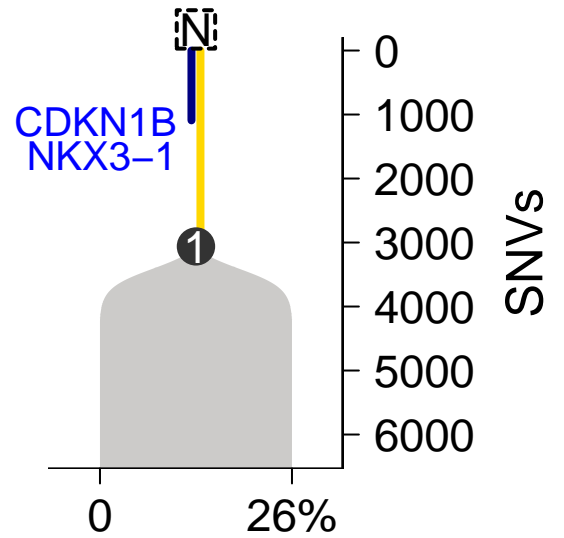
MuTect-TITAN
