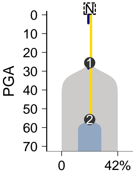
MuTect-Battenberg
