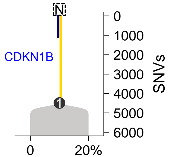
MuTect-TITAN
