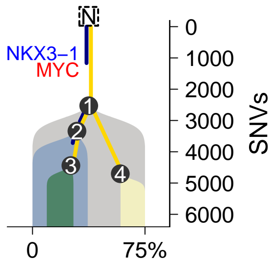
MuTect-TITAN
