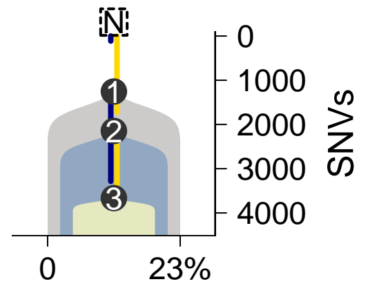
MuTect-TITAN
