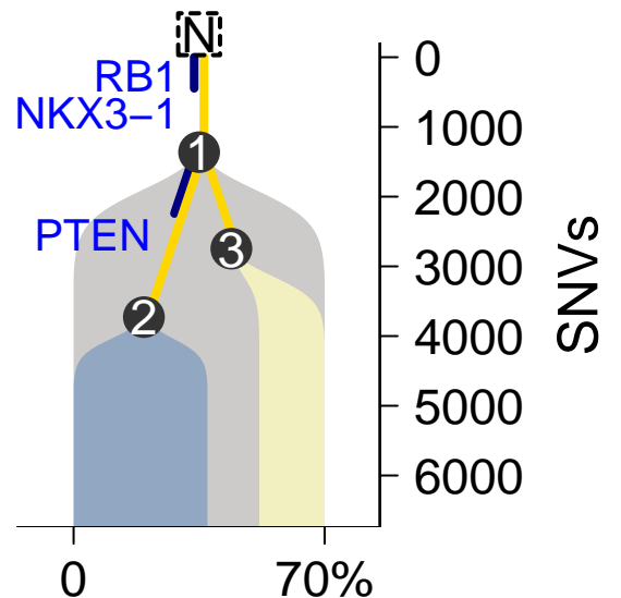
MuTect-TITAN
