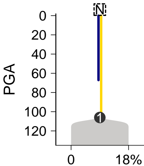
MuTect-Battenberg
