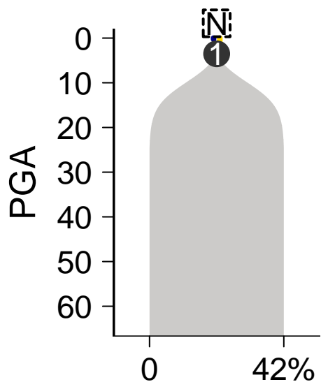
MuTect-Battenberg
