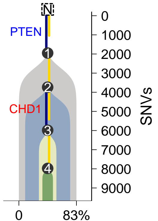
MuTect-TITAN
