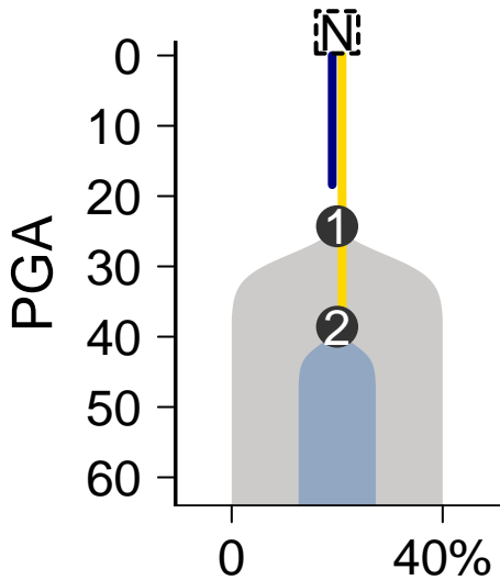
MuTect-Battenberg
