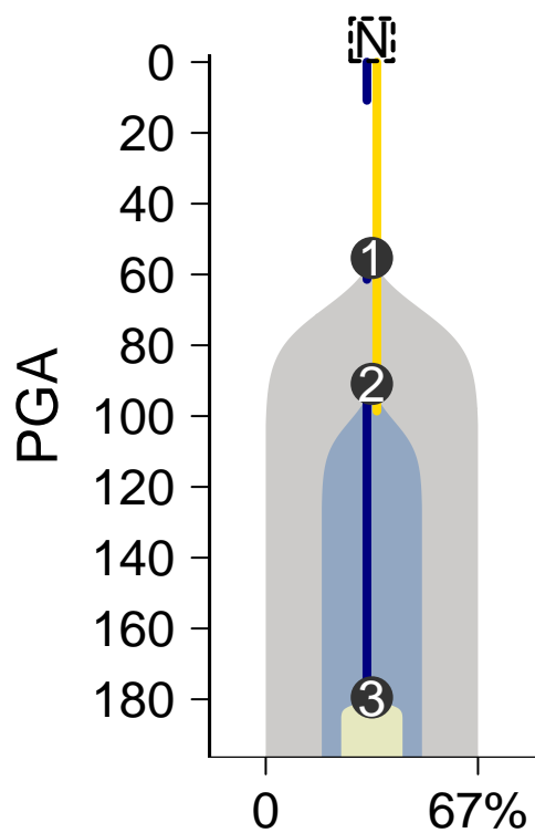
MuTect-Battenberg
