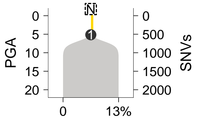
MuTect-TITAN
