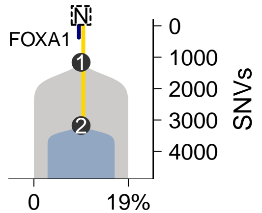
MuTect-TITAN
