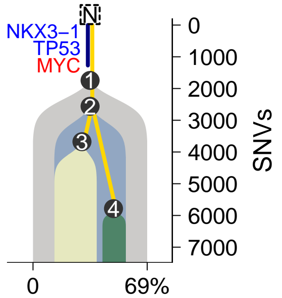
MuTect-TITAN
