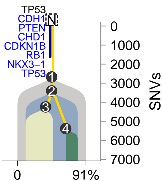
MuTect-TITAN
