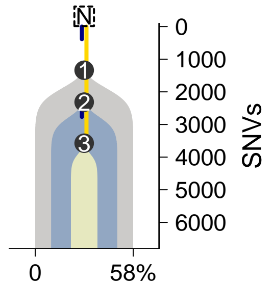
MuTect-TITAN
