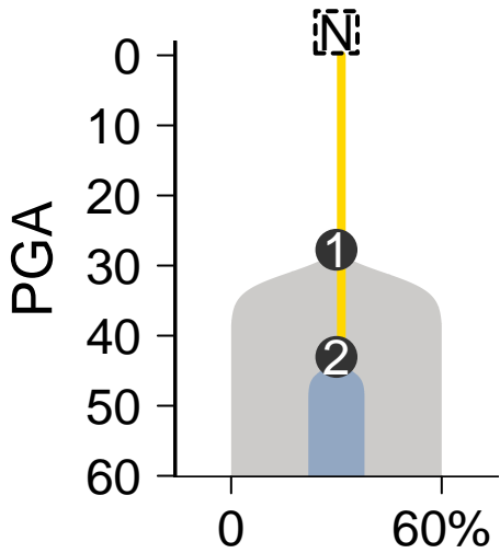
MuTect-Battenberg
