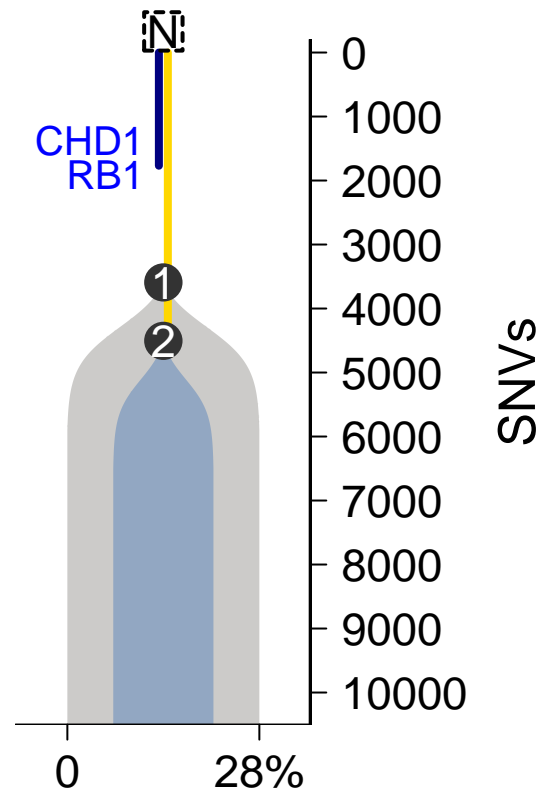
MuTect-TITAN
