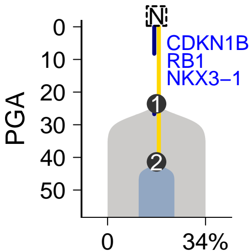
MuTect-Battenberg
