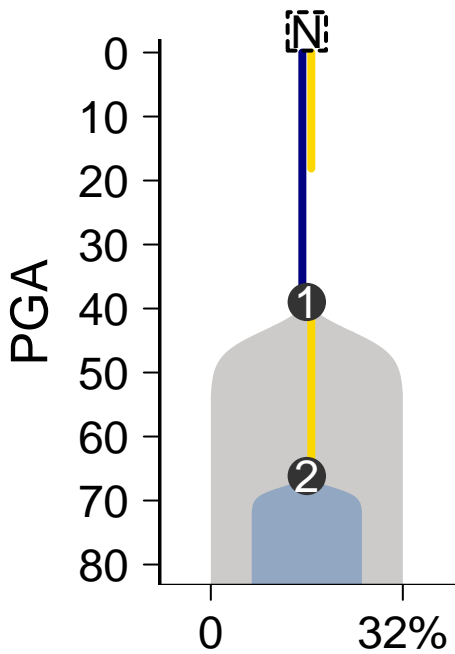
MuTect-Battenberg
