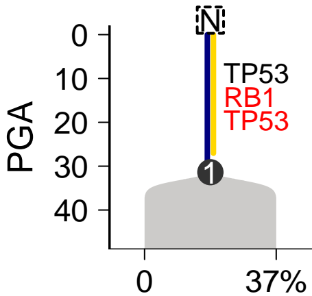
MuTect-Battenberg
