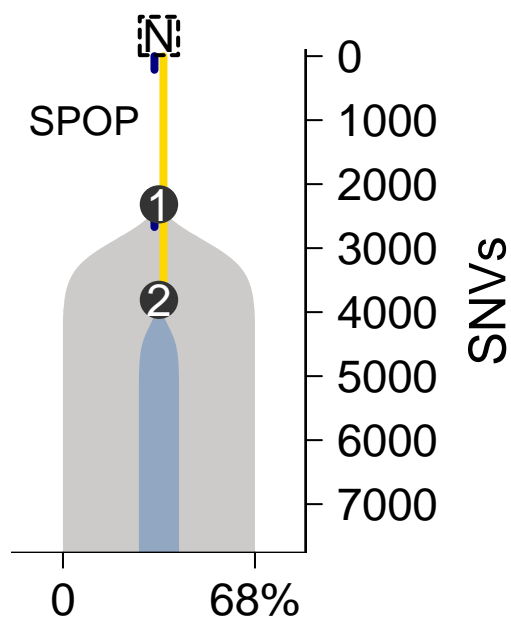
MuTect-TITAN
