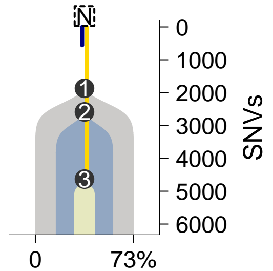
MuTect-TITAN
