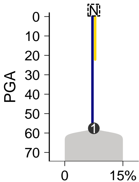
MuTect-Battenberg
