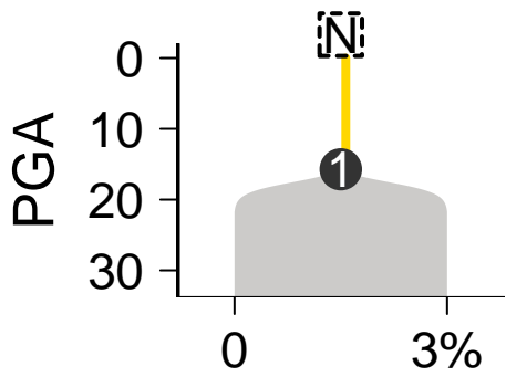
MuTect-Battenberg
