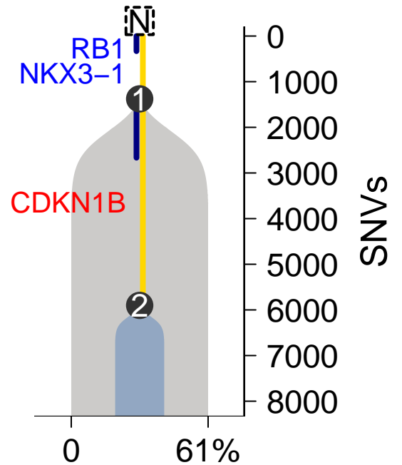
MuTect-TITAN
