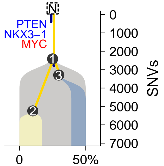
MuTect-TITAN
