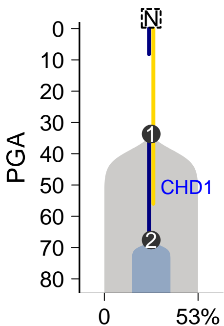
MuTect-Battenberg
