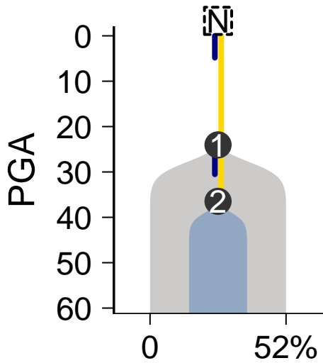
MuTect-Battenberg
