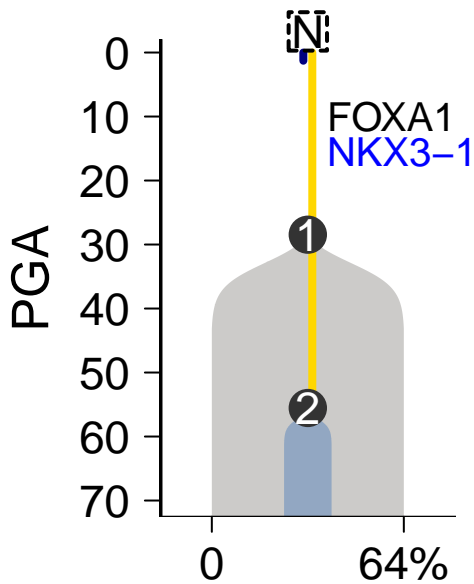
MuTect-Battenberg
