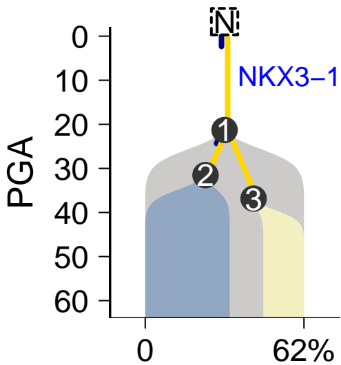
MuTect-Battenberg
