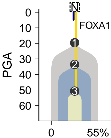
MuTect-Battenberg
