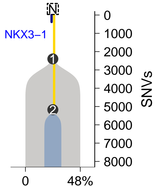
MuTect-TITAN
