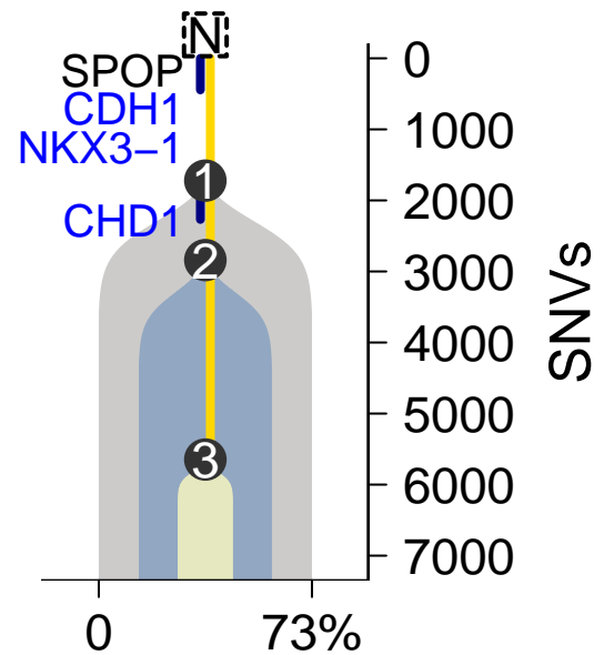
MuTect-TITAN
