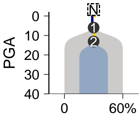
MuTect-Battenberg
