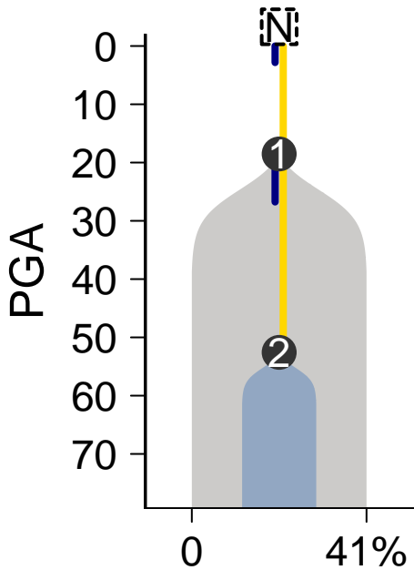
MuTect-Battenberg
