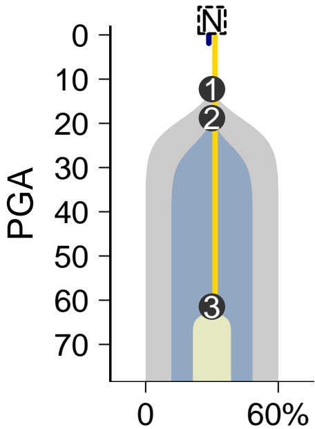
MuTect-Battenberg
