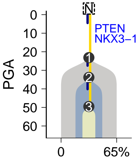
MuTect-Battenberg
