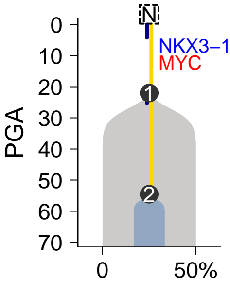
MuTect-Battenberg
