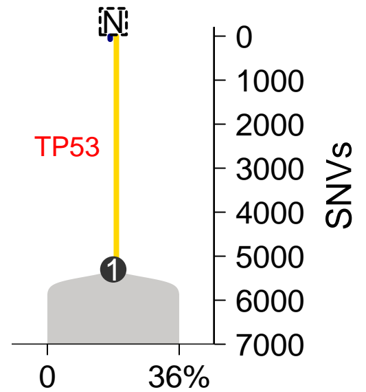
MuTect-TITAN
