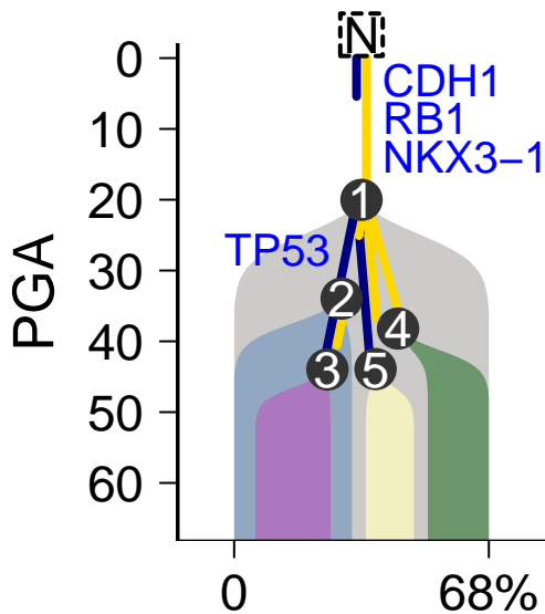
MuTect-Battenberg
