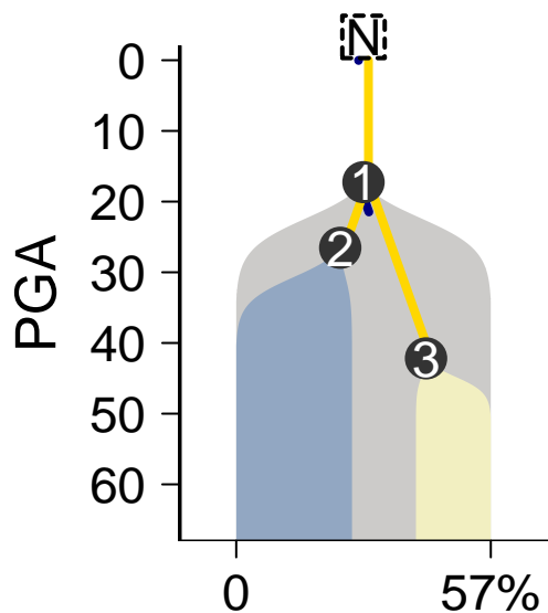
MuTect-Battenberg
