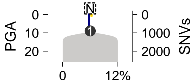
MuTect-TITAN
