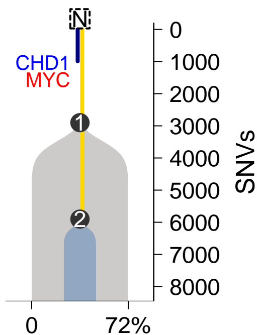
MuTect-TITAN
