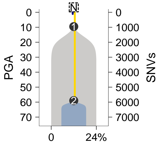
MuTect-TITAN
