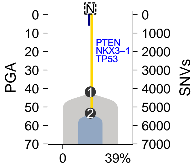
MuTect-TITAN
