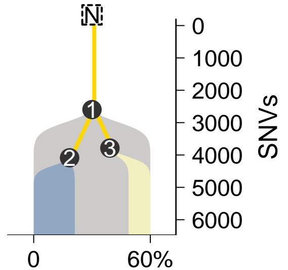
MuTect-TITAN
