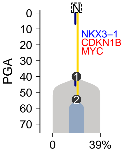
MuTect-Battenberg
