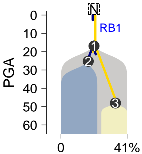
MuTect-Battenberg
