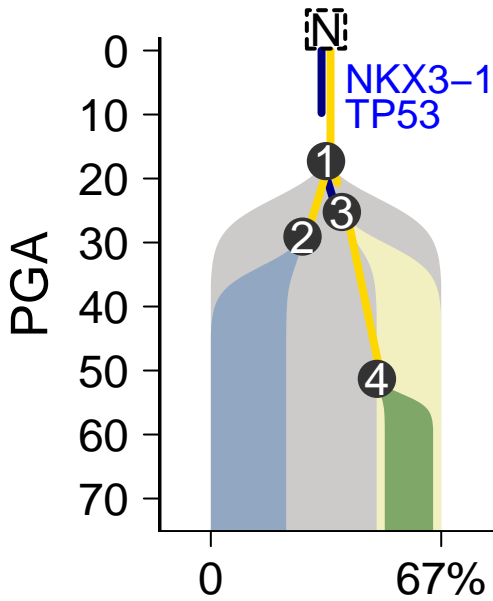
MuTect-Battenberg
