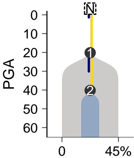
MuTect-Battenberg
