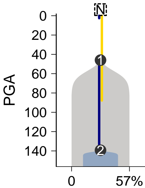
MuTect-Battenberg
