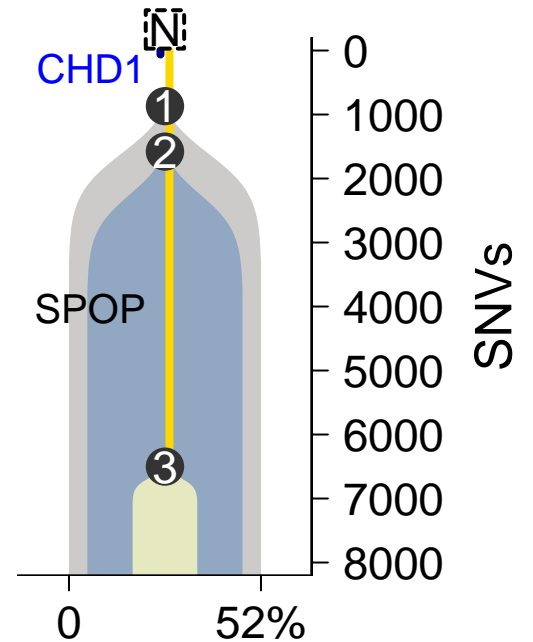
MuTect-TITAN
