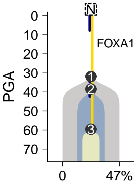
MuTect-Battenberg
