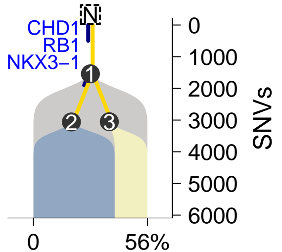
MuTect-TITAN
