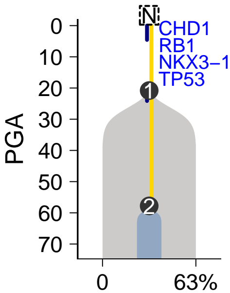
MuTect-Battenberg
