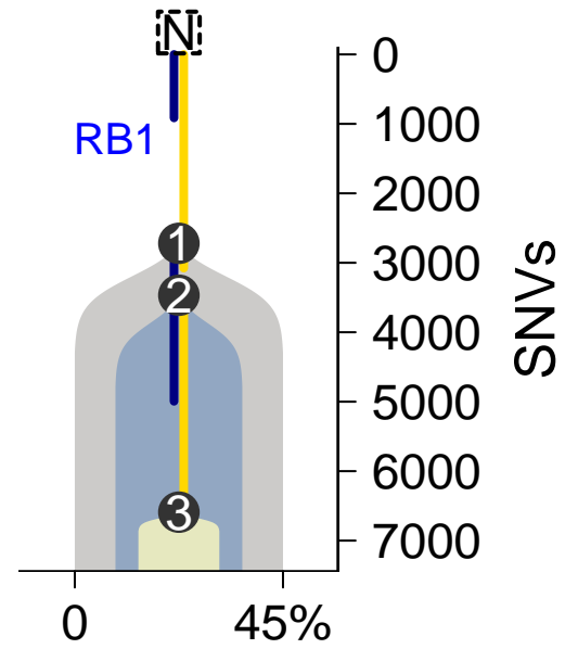
MuTect-TITAN
