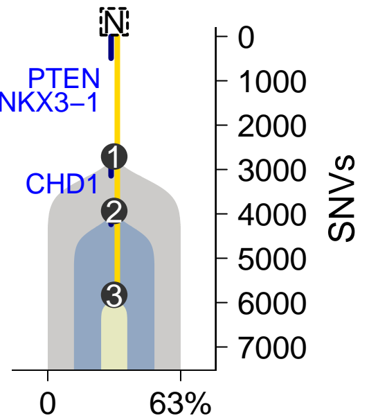
MuTect-TITAN
