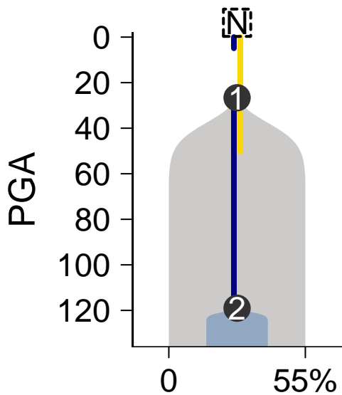
MuTect-Battenberg
