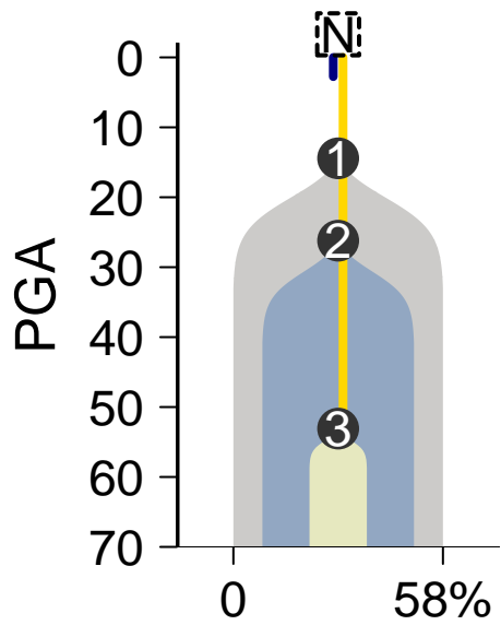
MuTect-Battenberg
