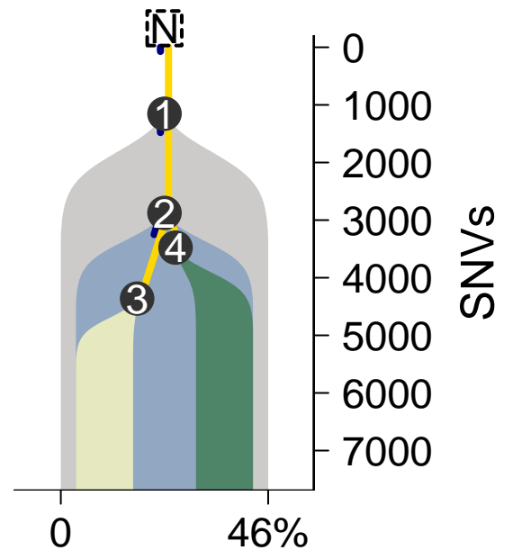
MuTect-TITAN
