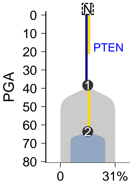
MuTect-Battenberg
