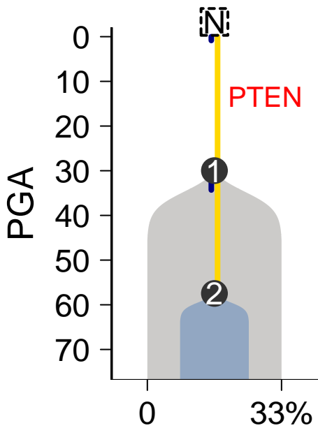
MuTect-Battenberg
