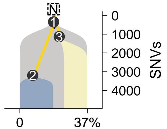
MuTect-TITAN
