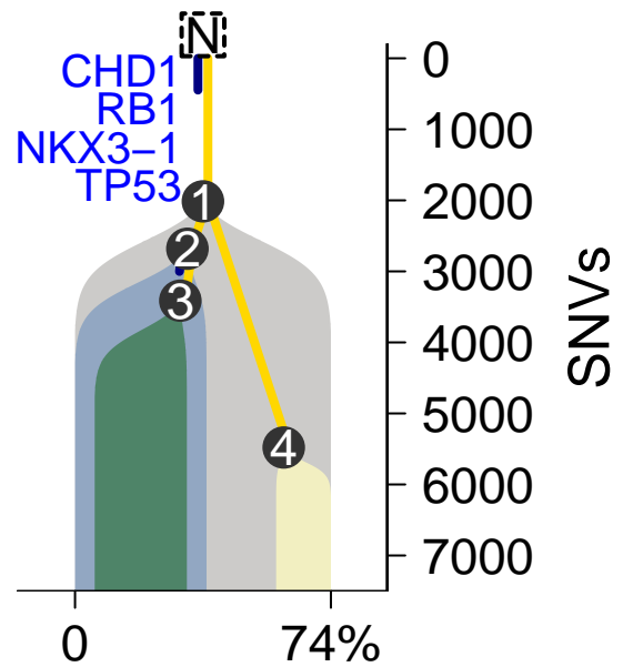
MuTect-TITAN
