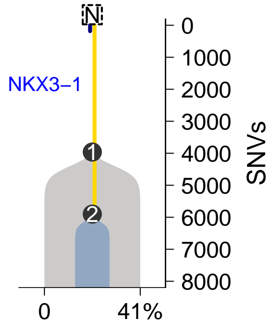
MuTect-TITAN
