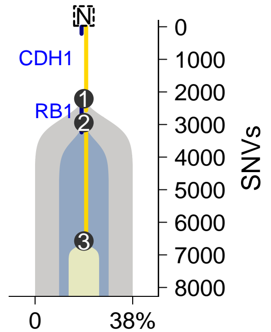
MuTect-TITAN
