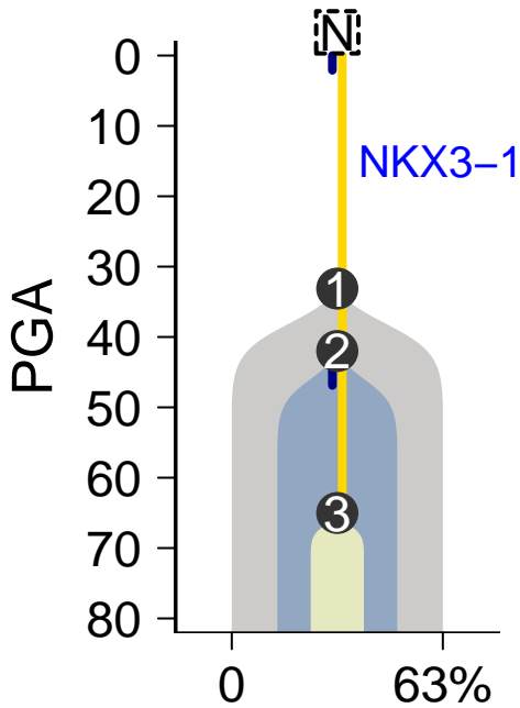
MuTect-Battenberg
