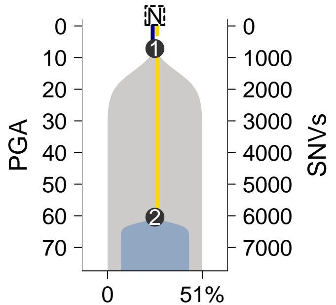
MuTect-TITAN
