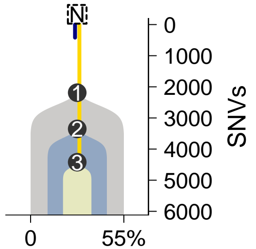
MuTect-TITAN
