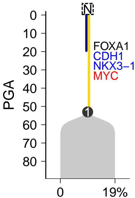
MuTect-Battenberg
