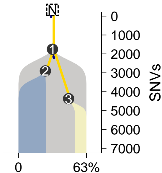
MuTect-TITAN
