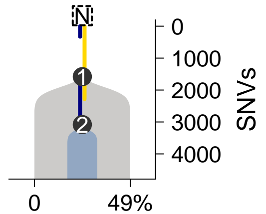
MuTect-TITAN
