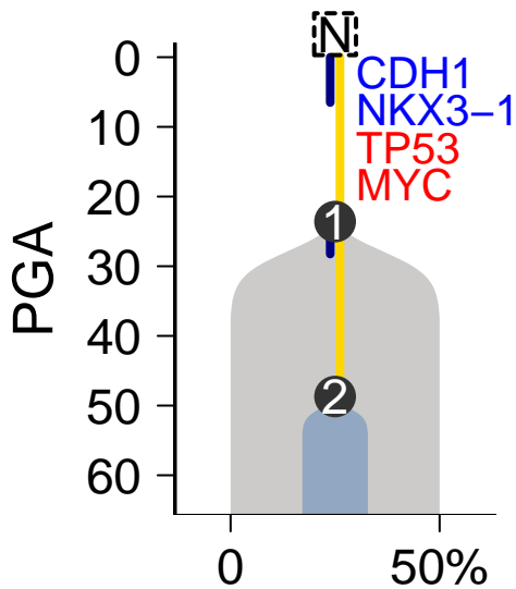
MuTect-Battenberg
