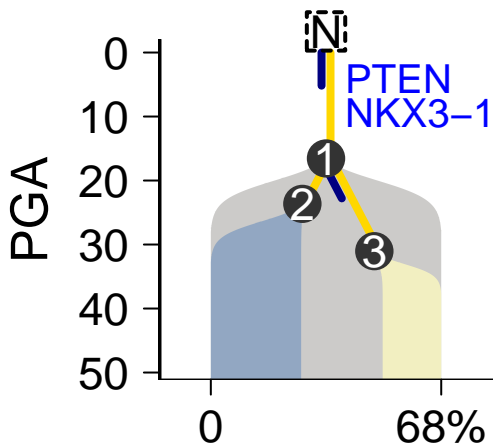
MuTect-Battenberg
