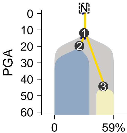
MuTect-Battenberg
