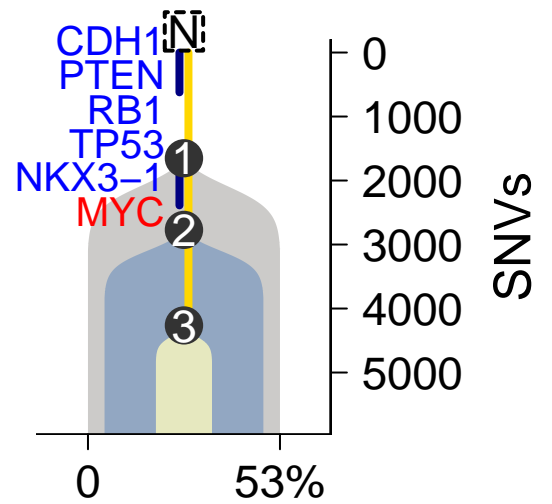
MuTect-TITAN
