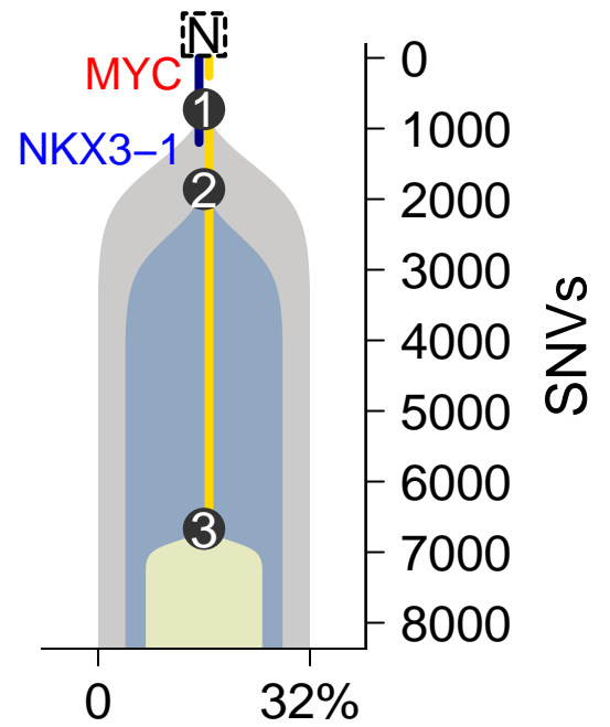
MuTect-TITAN
