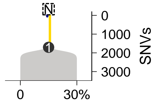
MuTect-TITAN
