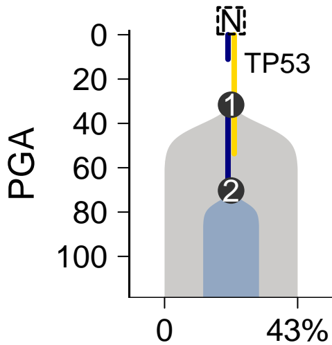
MuTect-Battenberg
