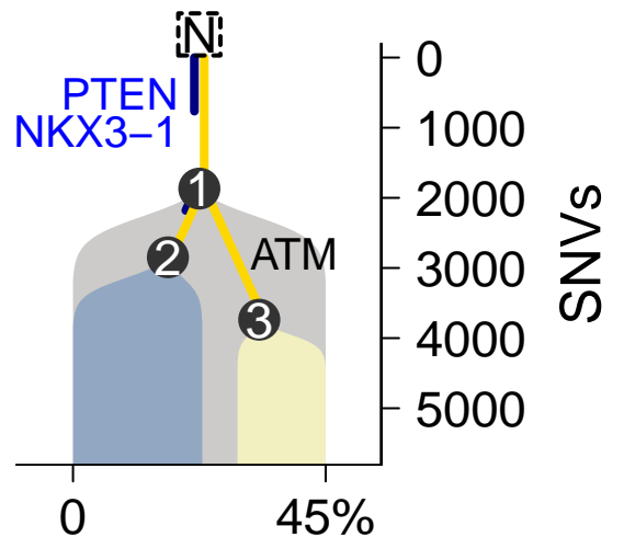
MuTect-TITAN
