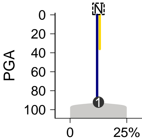
MuTect-Battenberg
