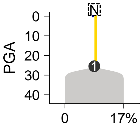
MuTect-Battenberg
