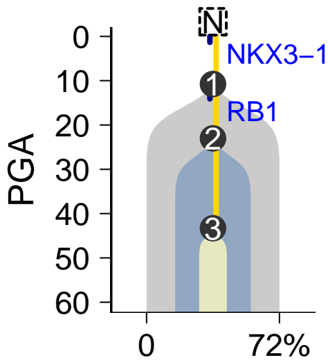
MuTect-Battenberg
