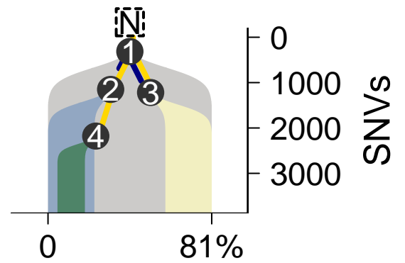
MuTect-TITAN
