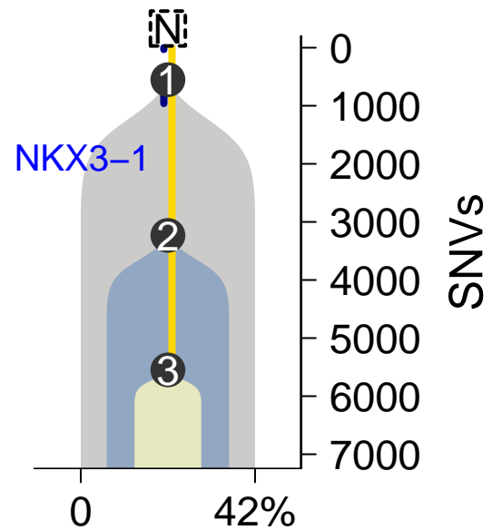
MuTect-TITAN
