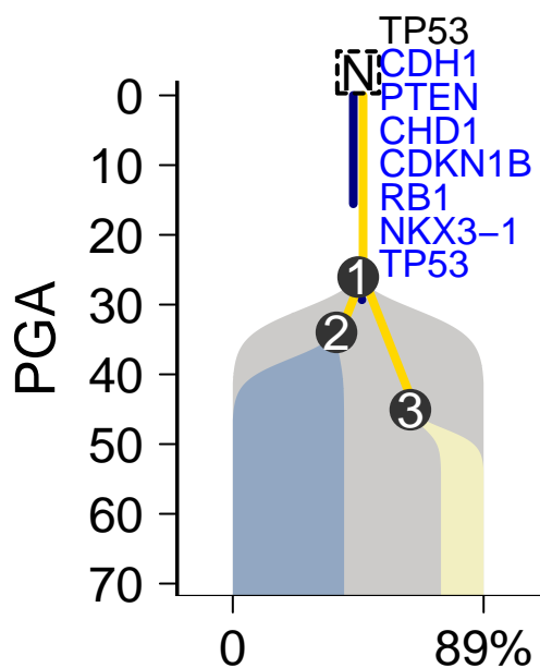
MuTect-Battenberg
