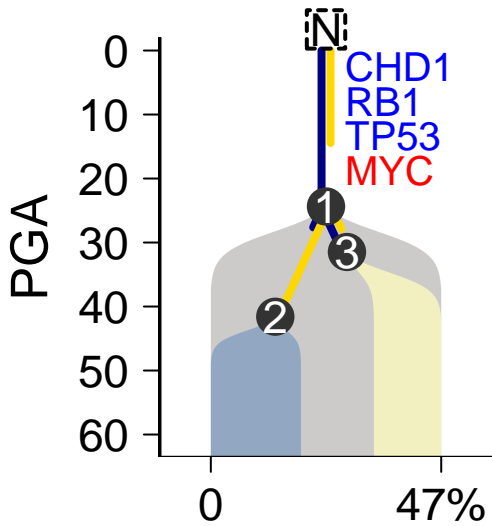
MuTect-Battenberg
