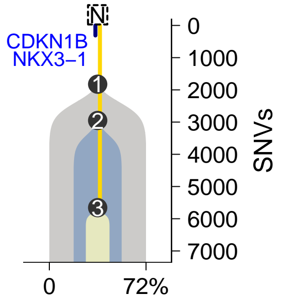
MuTect-TITAN
