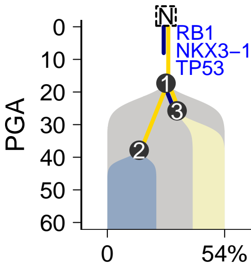
MuTect-Battenberg
