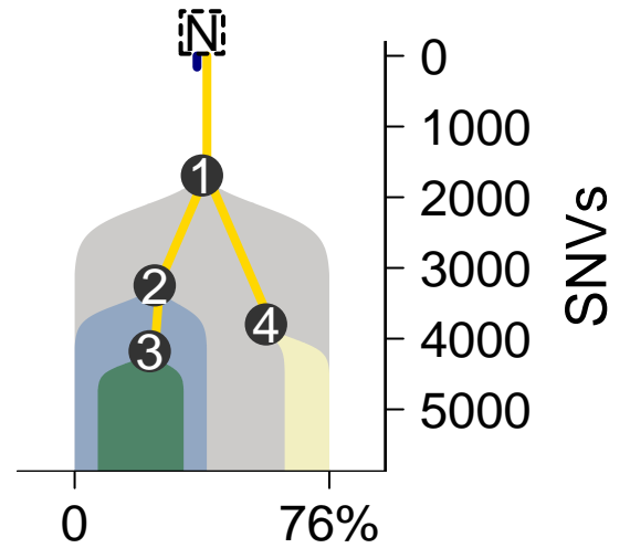
MuTect-TITAN
