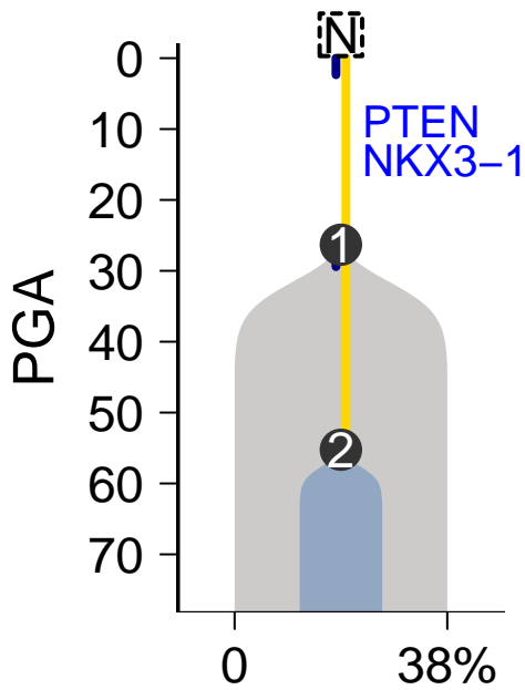
MuTect-Battenberg
