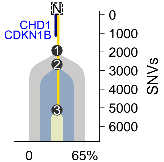
MuTect-TITAN
