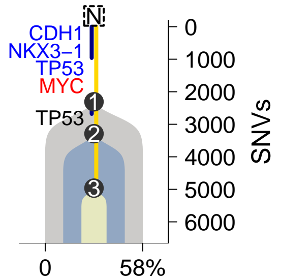
MuTect-TITAN
