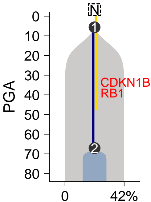
MuTect-Battenberg
