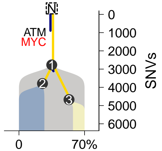
MuTect-TITAN
