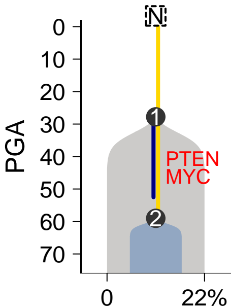
MuTect-Battenberg
