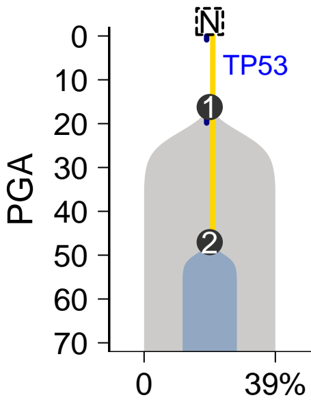
MuTect-Battenberg
