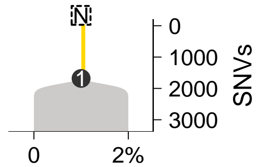
MuTect-TITAN
