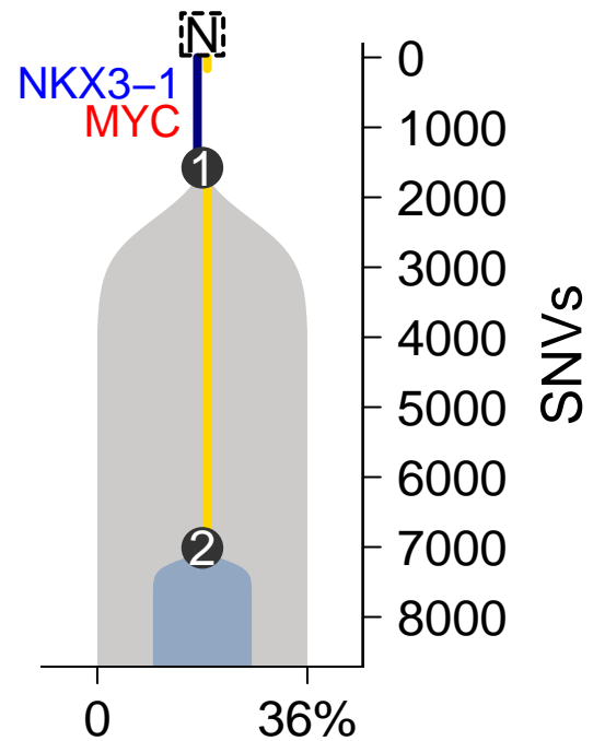
MuTect-TITAN
