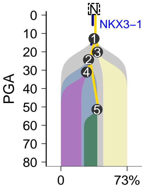
MuTect-Battenberg
