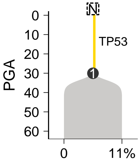
MuTect-Battenberg
