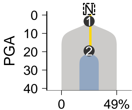
MuTect-Battenberg
