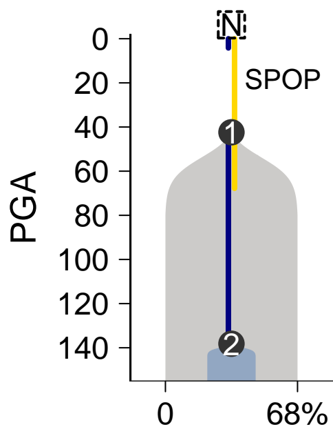
MuTect-Battenberg
