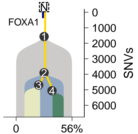
MuTect-TITAN
