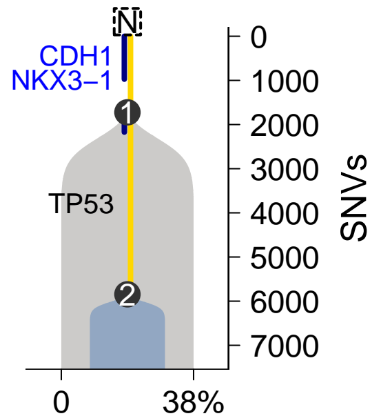
MuTect-TITAN
