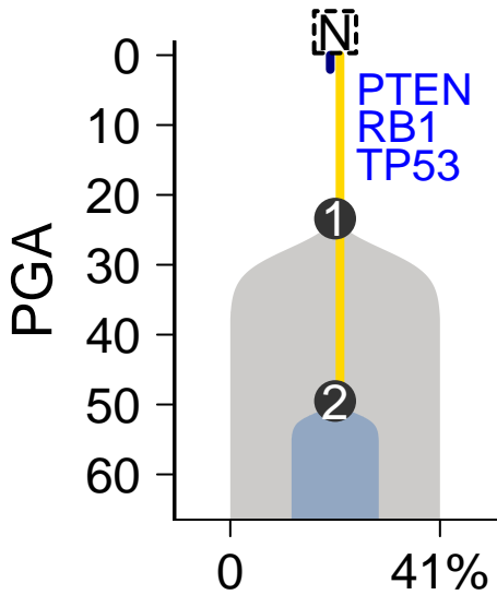
MuTect-Battenberg
