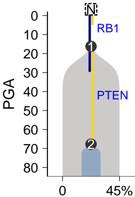
MuTect-Battenberg
