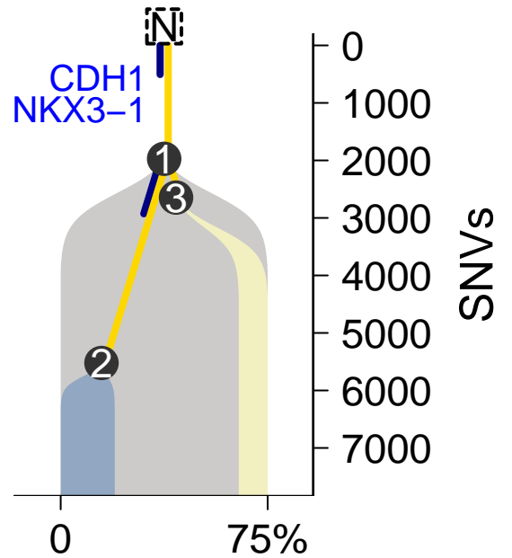
MuTect-TITAN
