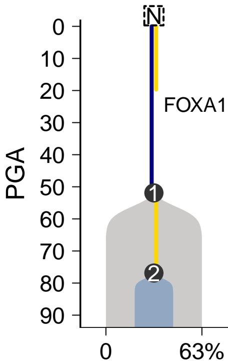
MuTect-Battenberg
