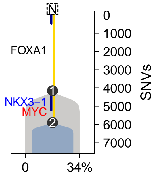
MuTect-TITAN
