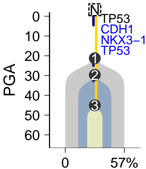
MuTect-Battenberg
