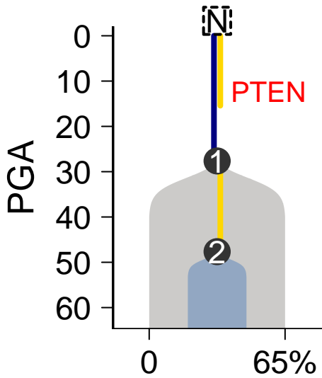
MuTect-Battenberg
