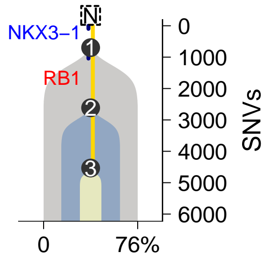
MuTect-TITAN
