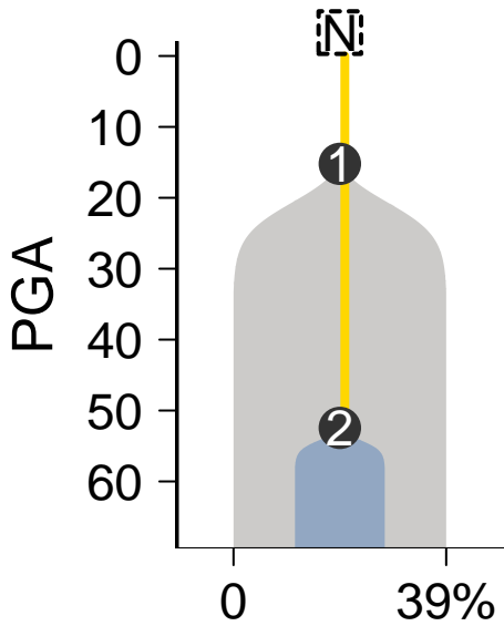
MuTect-Battenberg
