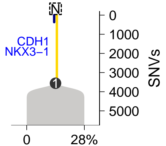
MuTect-TITAN
