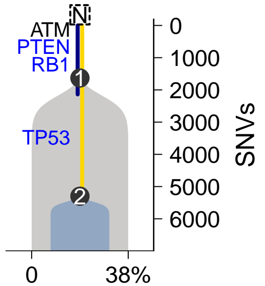
MuTect-TITAN
