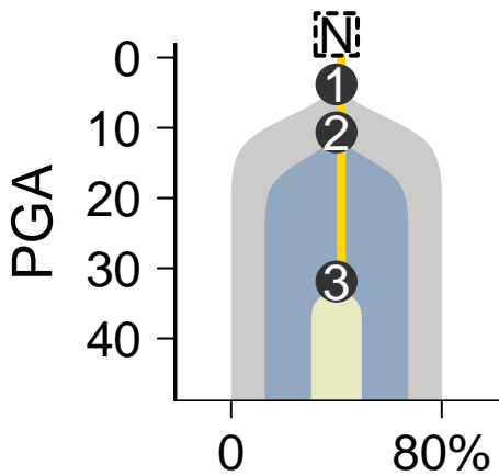
MuTect-Battenberg
