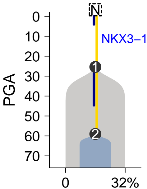
MuTect-Battenberg
