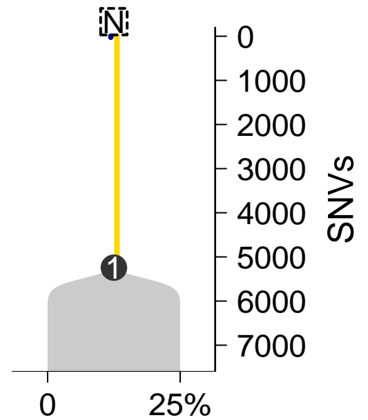
MuTect-TITAN
