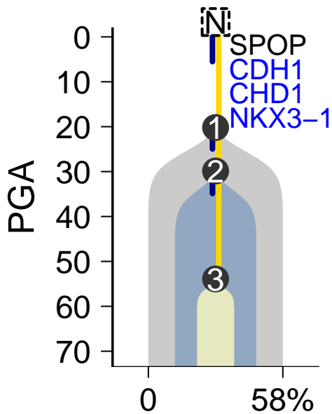
MuTect-Battenberg
