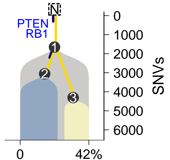
MuTect-TITAN
