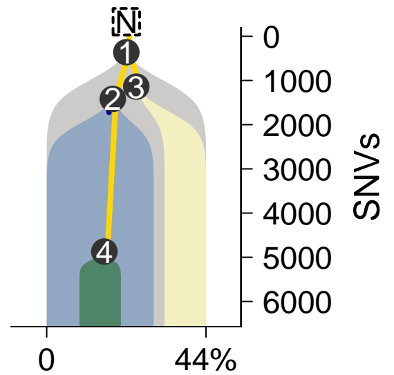
MuTect-TITAN
