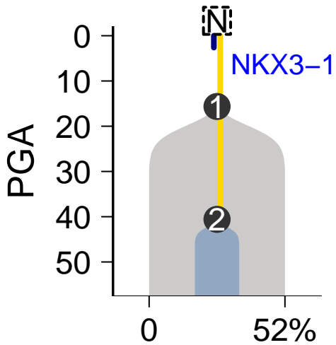
MuTect-Battenberg
