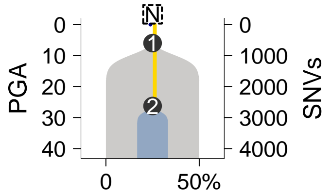
MuTect-TITAN
