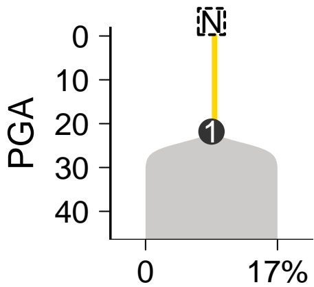
MuTect-Battenberg
