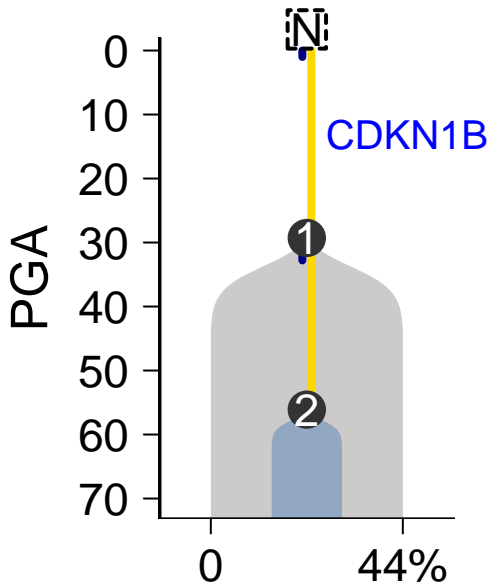
MuTect-Battenberg
