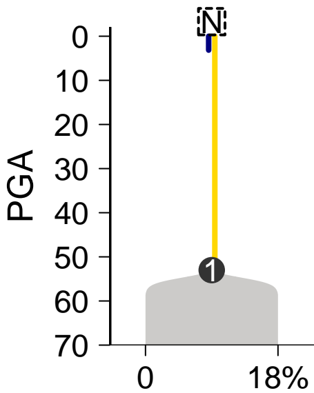
MuTect-Battenberg
