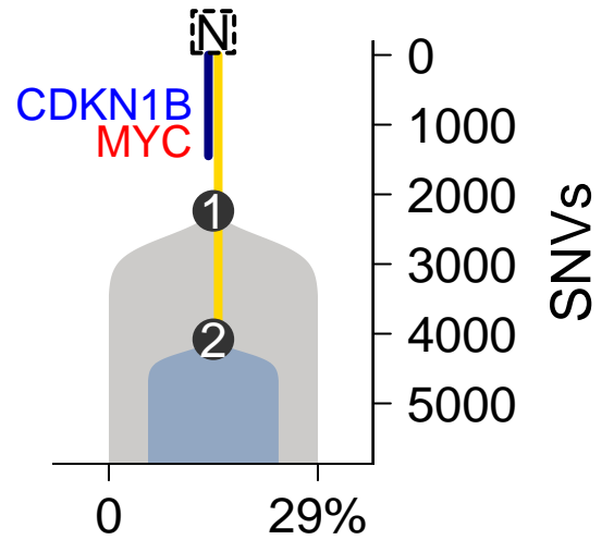
MuTect-TITAN
