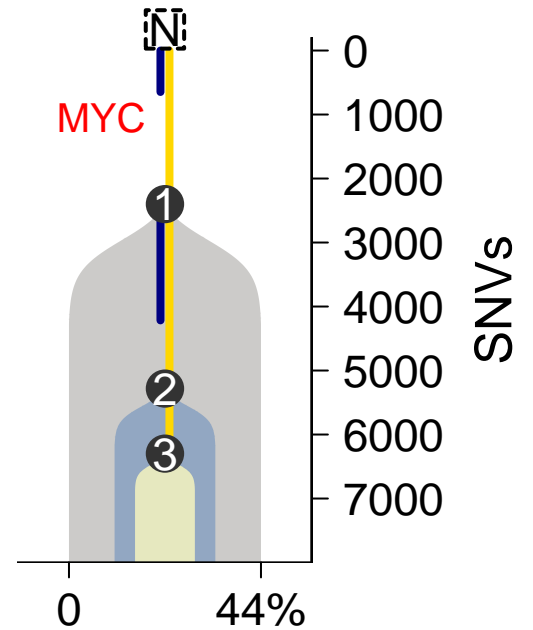
MuTect-TITAN
