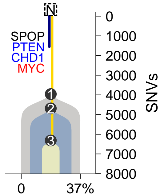
MuTect-TITAN
