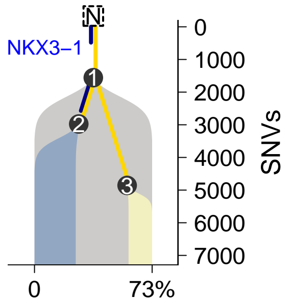
MuTect-TITAN
