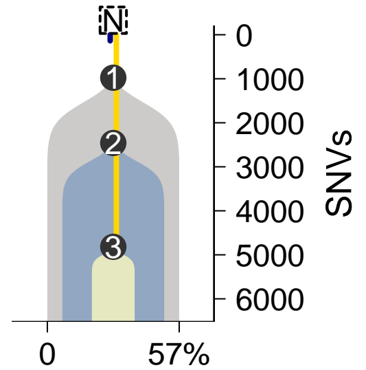
MuTect-TITAN
