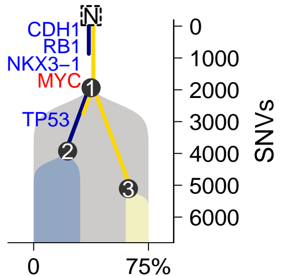
MuTect-TITAN
