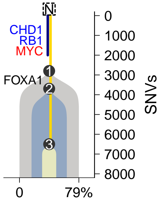
MuTect-TITAN
