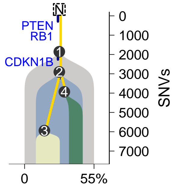
MuTect-TITAN
