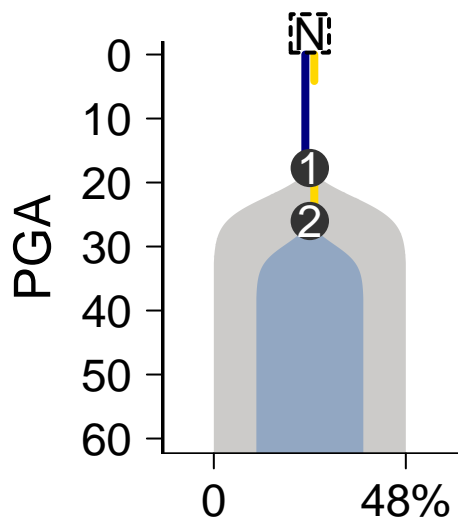
MuTect-Battenberg
