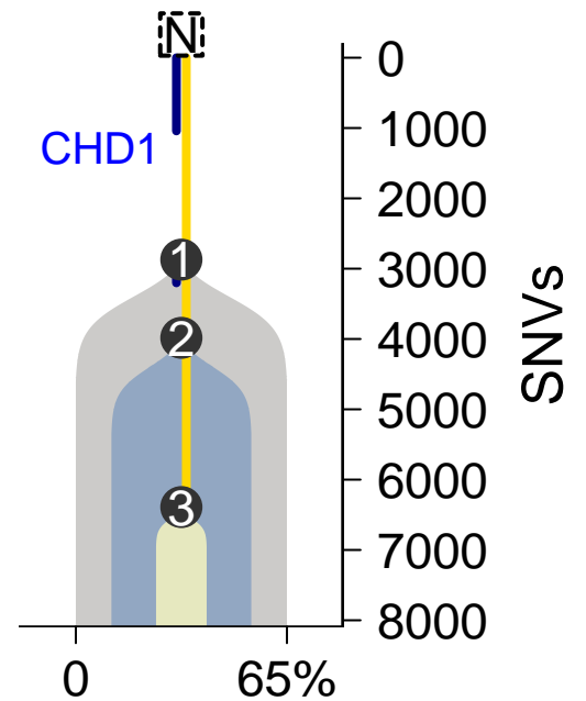
MuTect-TITAN
