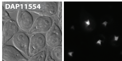
DAP11554 Nek kinase
