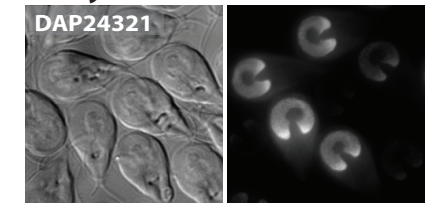
Nek kinase
